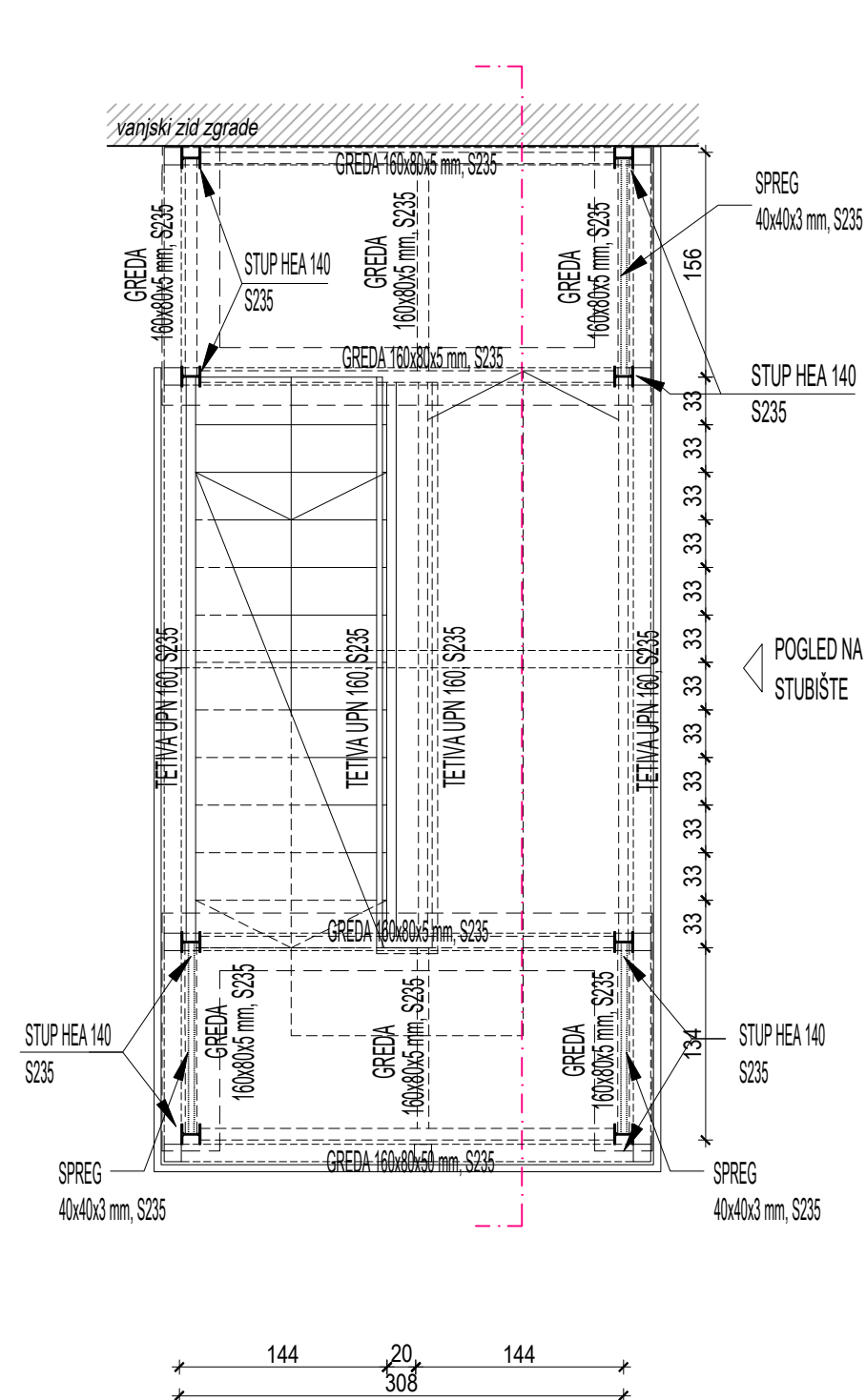
TLOCRT PRIZEMLJA
