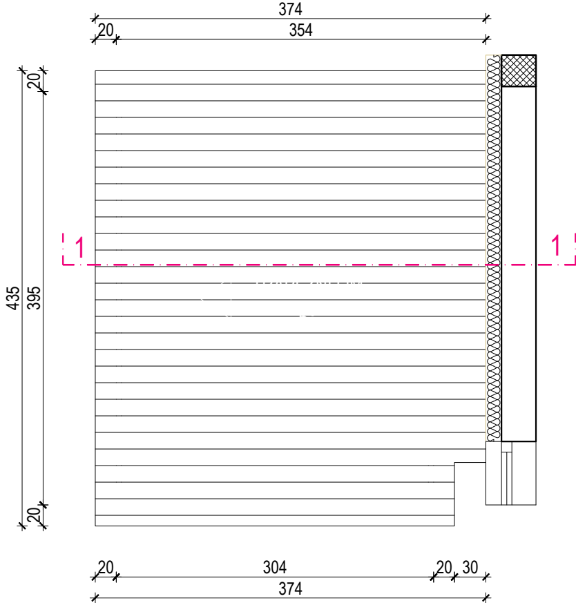
TLOCRT KROVNIH PLOHA
