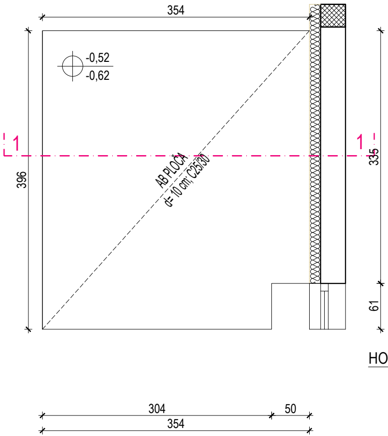
TLOCRT TEMELJA
