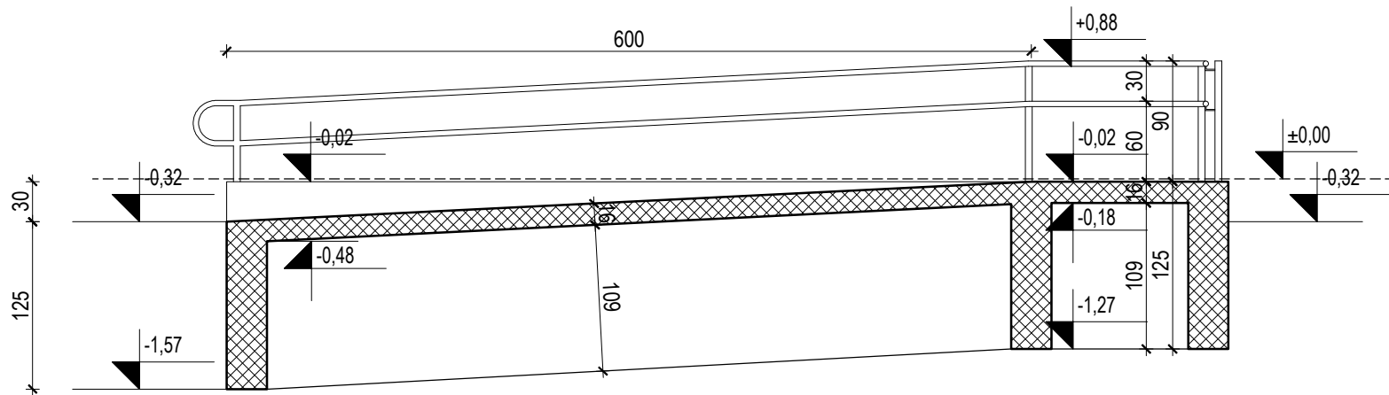
PRESJEK A-A
