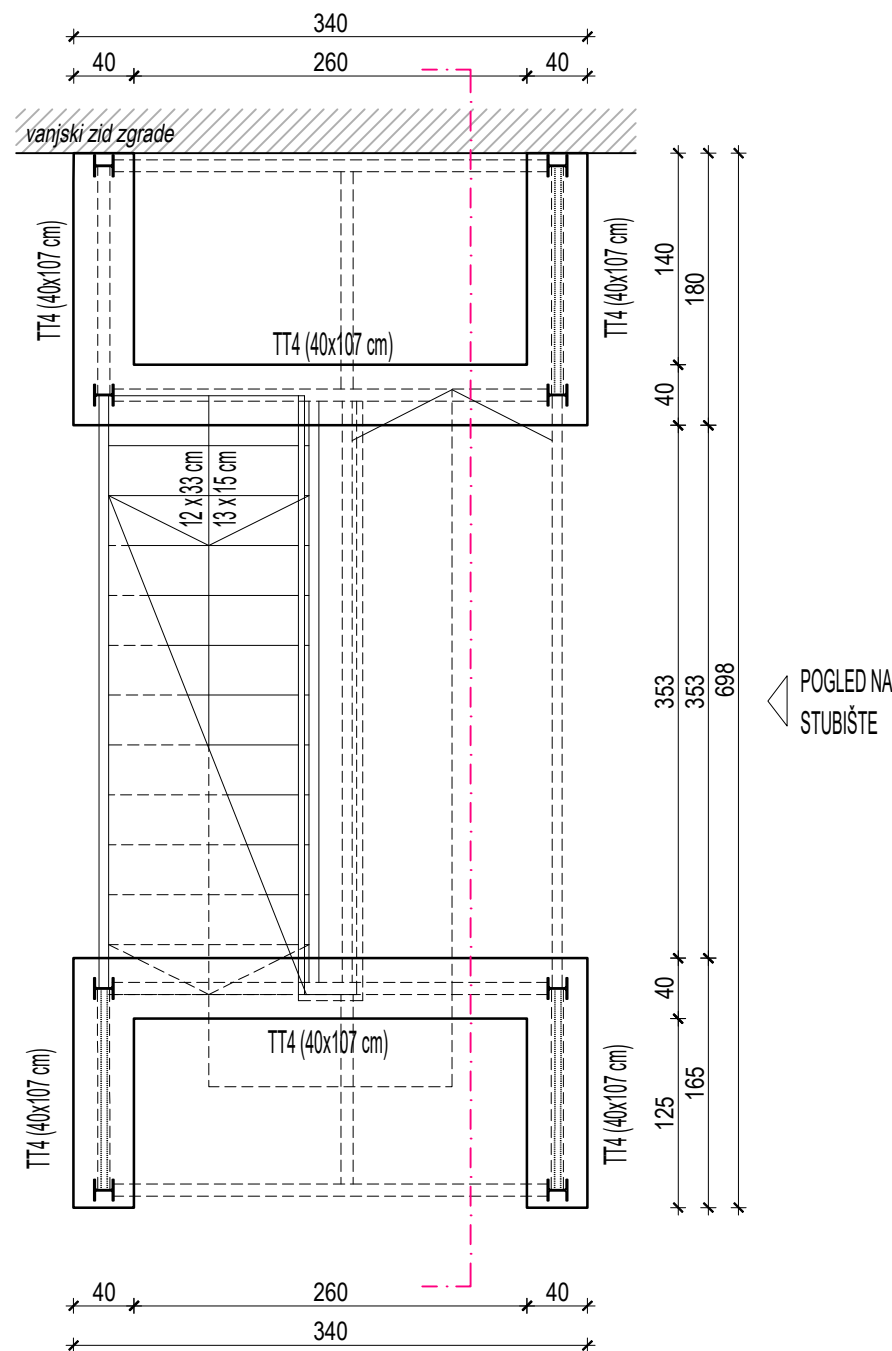
TLOCRT TEMELJA
