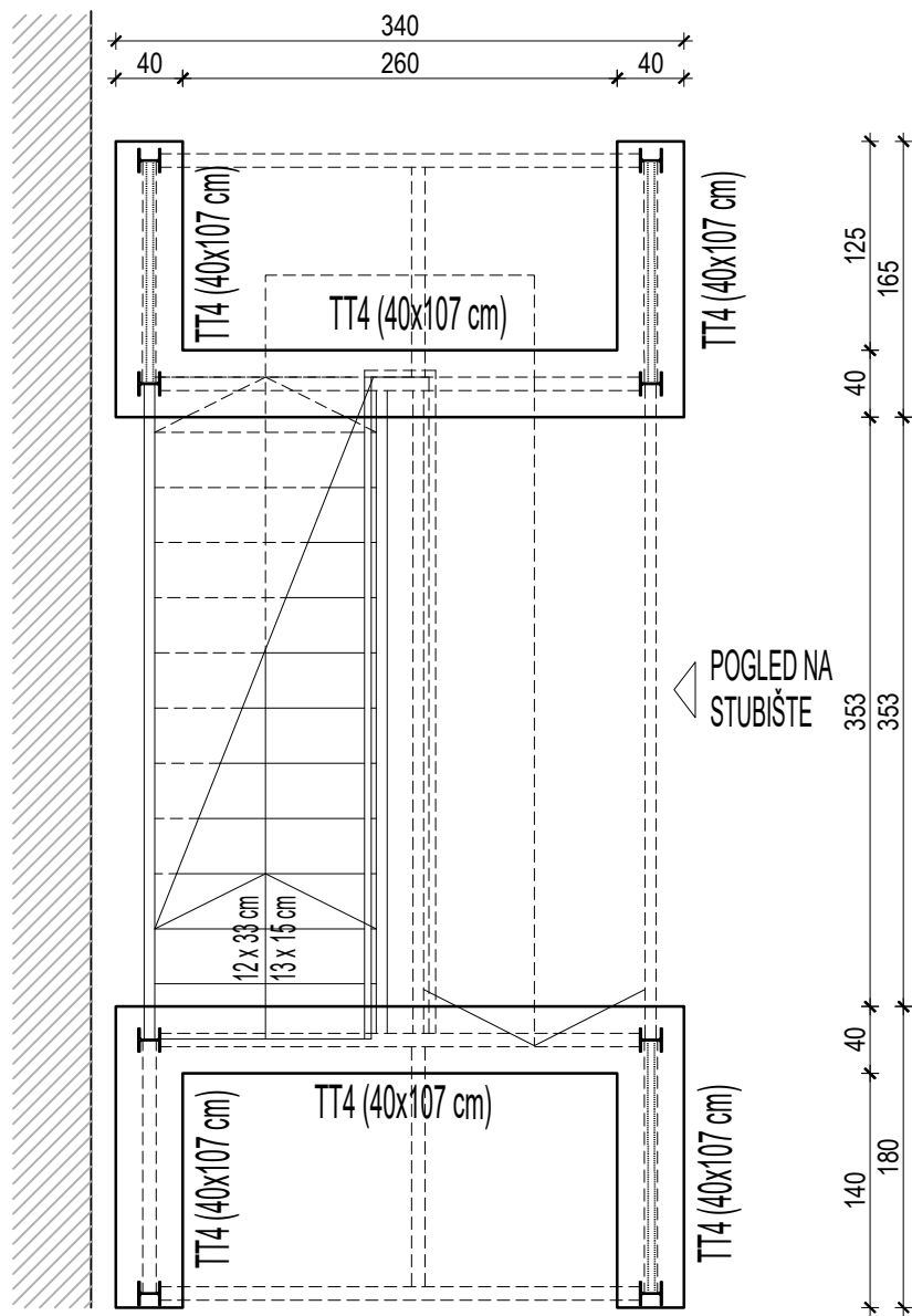
TLOCRT TEMELJA
