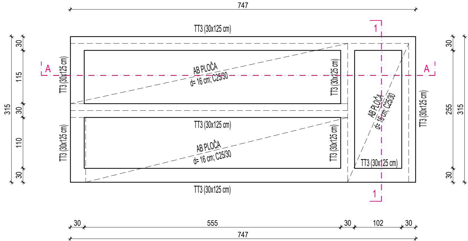
TLOCRT TEMELJA
