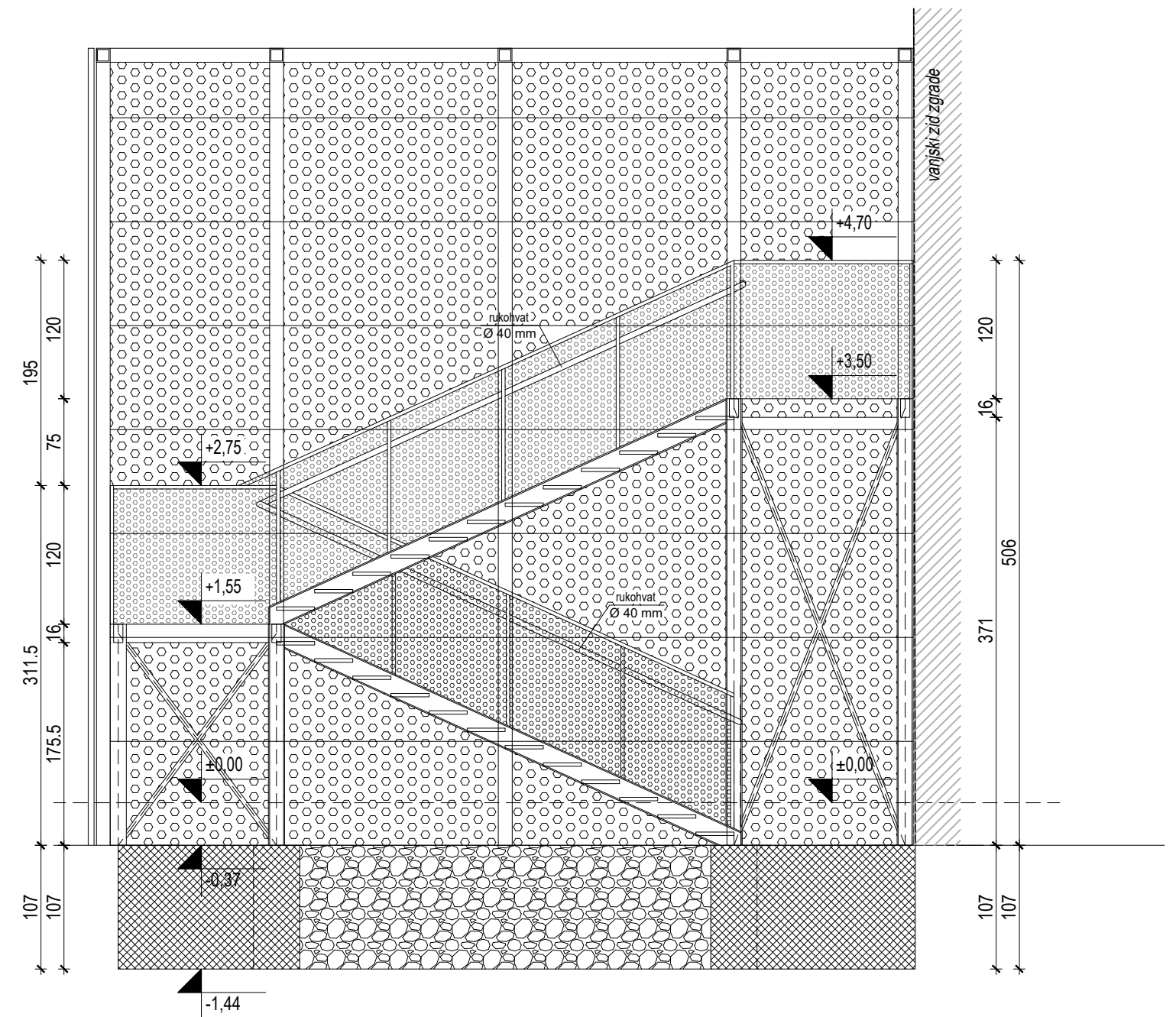
UZDUŽNI PRESJEK
