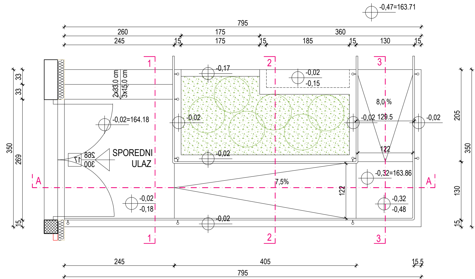
TLOCRT PRIZEMLJA
