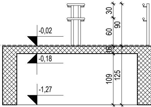
PRESJEK 1-1
