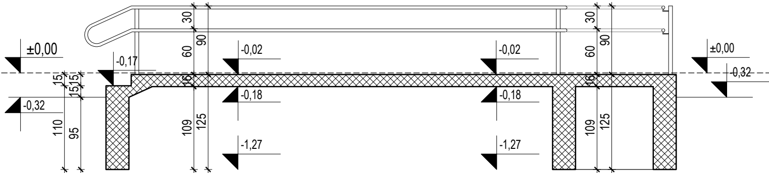
PRESJEK B-B
