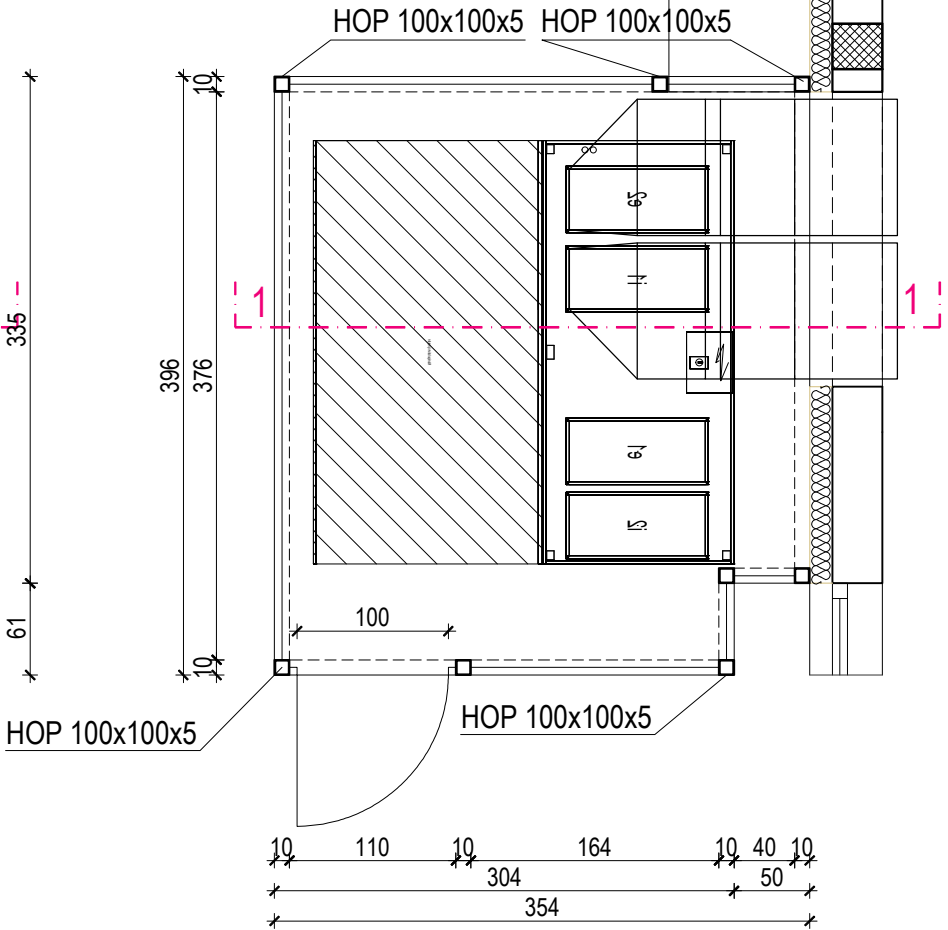
TLOCRT PRIZEMLJA
