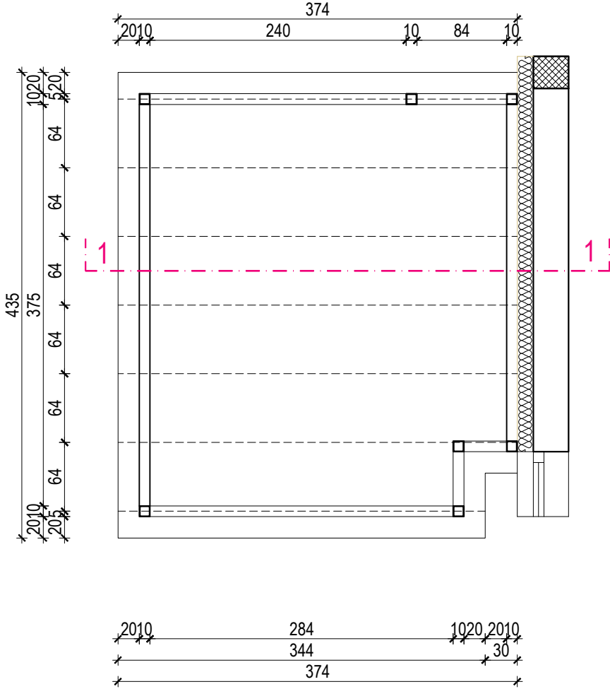
TLOCRT KROVNE KONSTRUKCIJE
