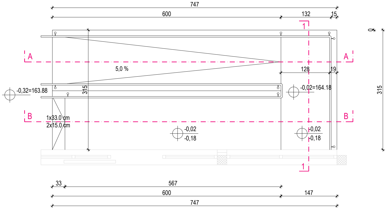
TLOCRT PRIZEMLJA
