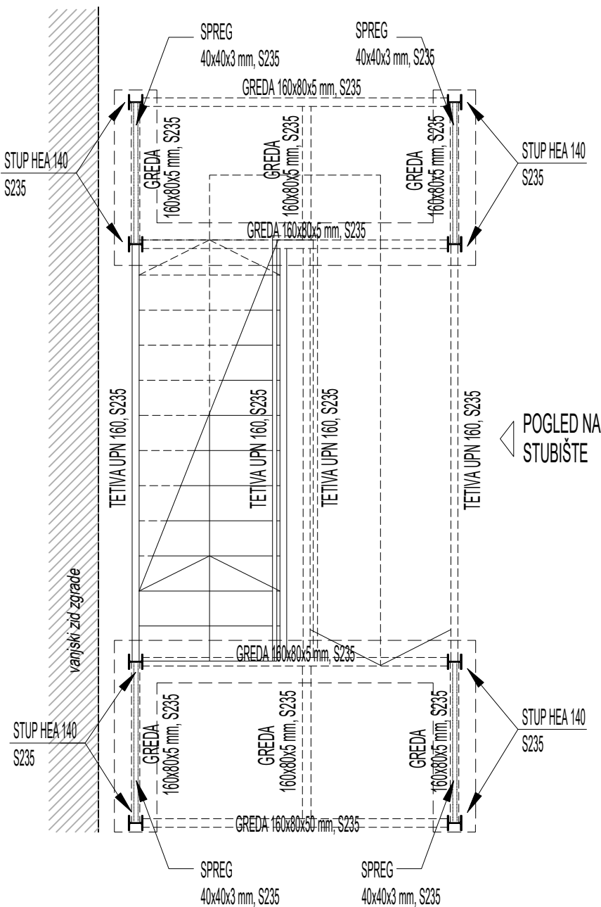
TLOCRT PRIZEMLJA
