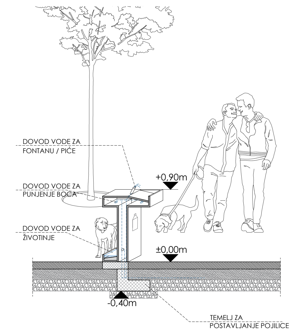
DETALJ / PITKA VODA M 1:30
