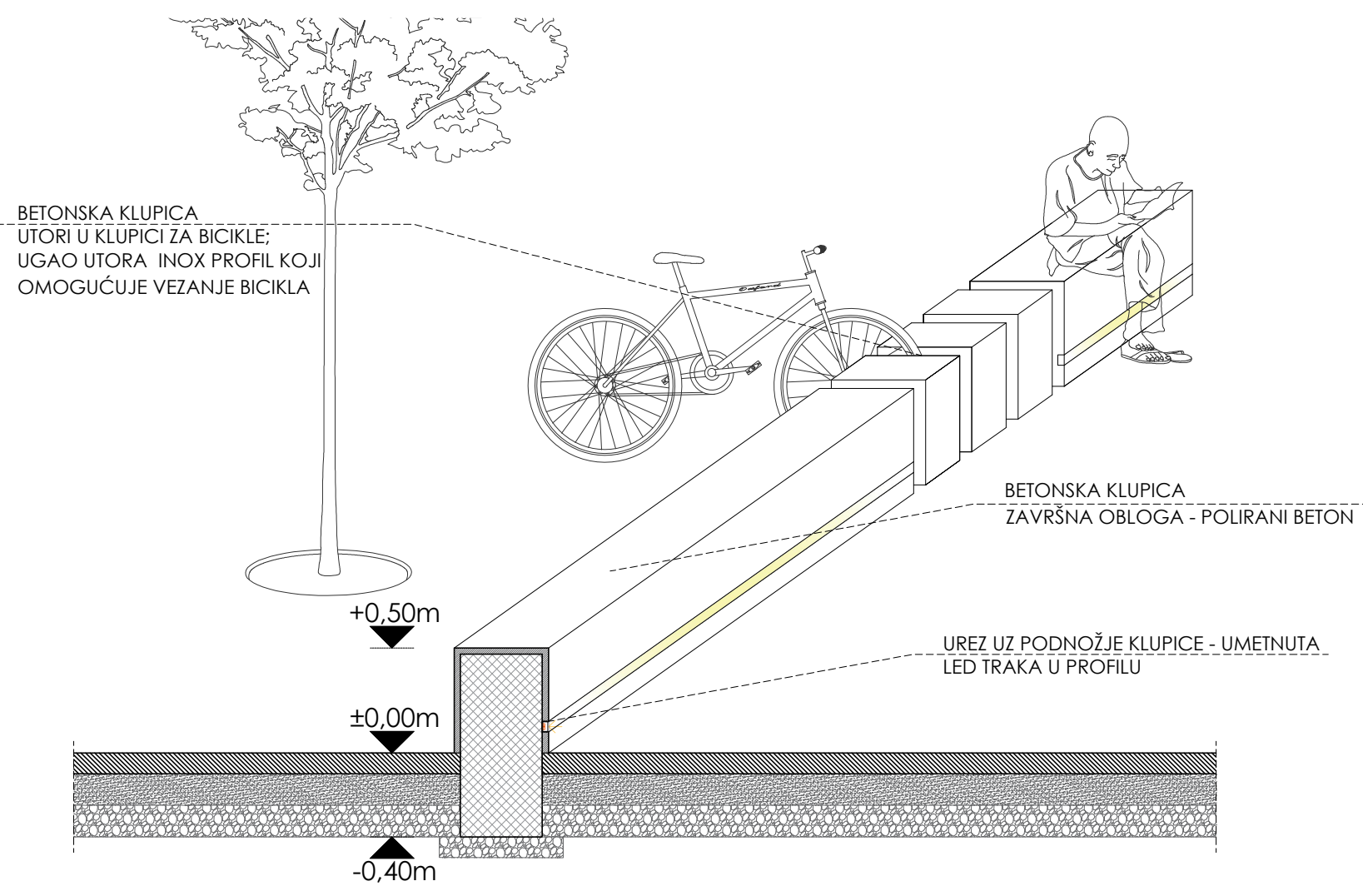
DETALJ / KLUPICA M 1:30
