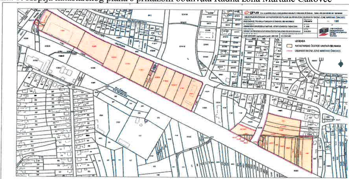
Slika 1: Kopija katastarskog plana s prikazom obuhvata Radna zona Martane Čakovec
